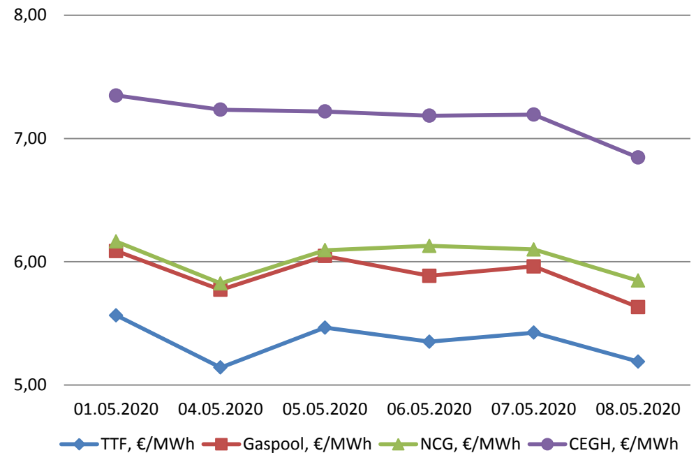
Графік 2. Спотові котирування на природний газ на європейських хабах TTF, Gaspool, NCG, CEGH, €/MWh
